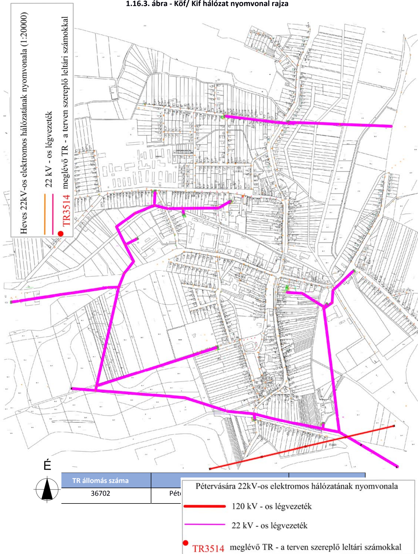
1.16.3. ábra - Köf/ Kif hálózat nyomvonal rajza
