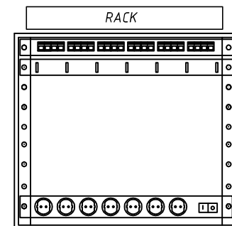
Szekrény mérete: 9U A szekrényben az aktív eszközöket a választott gyá. szolgáltató helyezi el.
