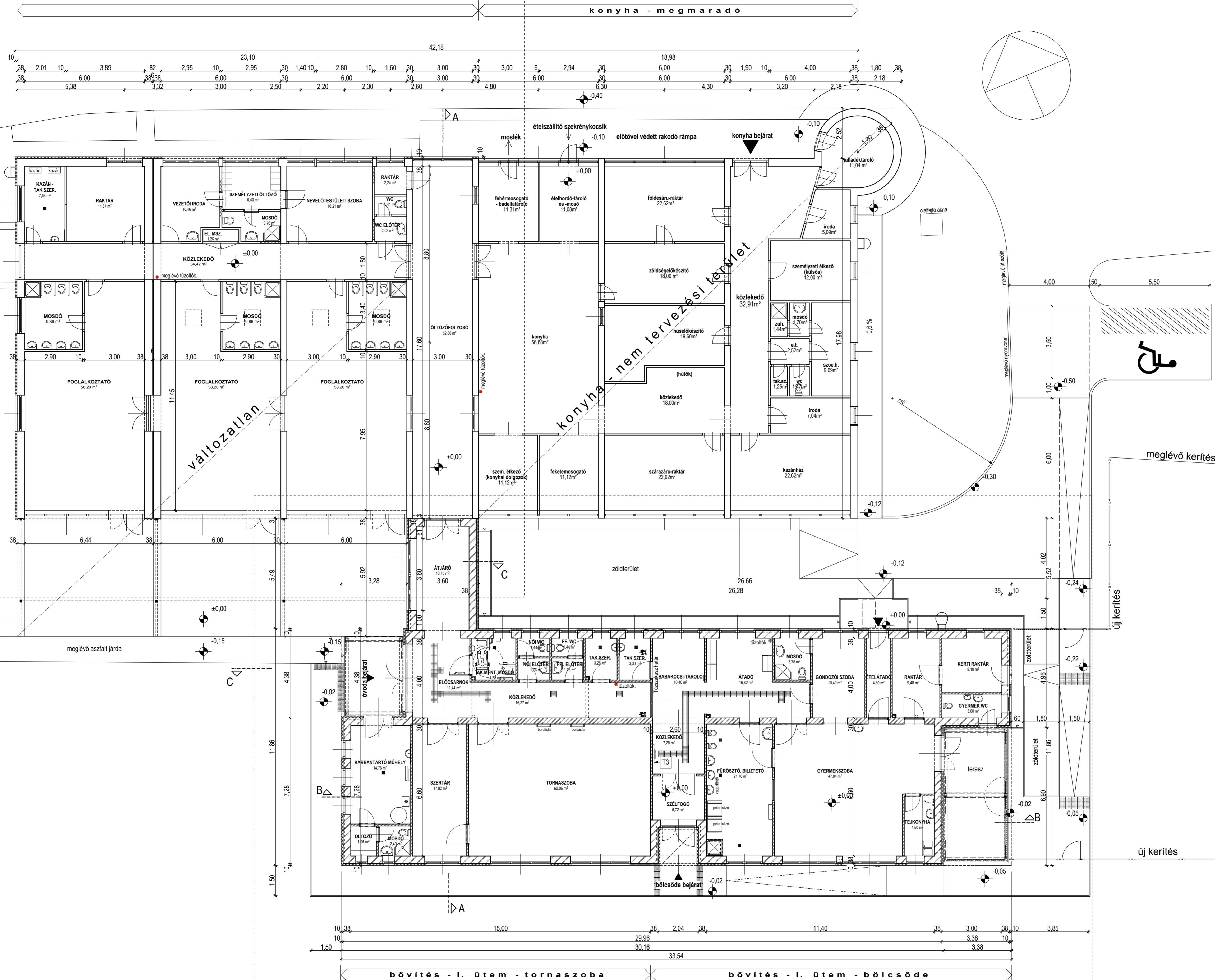
E - 01 / B Bővítési alaprajz
